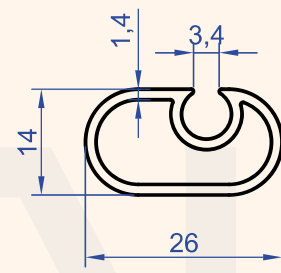
Profil No : 1267 Gramaj : 0.287 kg/m
