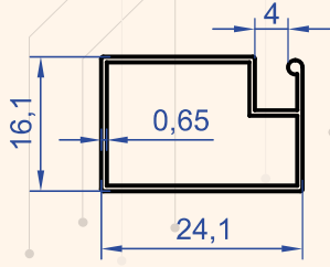
Profil No : 1194 Gramaj : 0.149 kg/m
