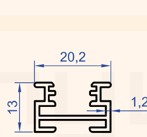
Profil No : 7967 Gramaj : 0.223 kg/m
