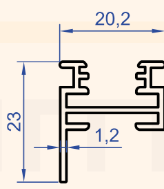
Profil No : 7968 Gramaj : 0.255 kg/m
