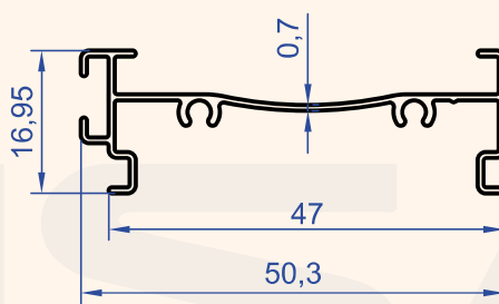
Profil No : 2027 Gramaj : 0.236 kg/m
