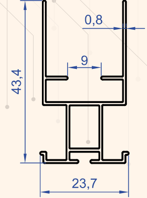
Profil No : 2134 Gramaj : 0.330 kg/m
