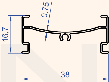
Profil No : 2028 Gramaj : 0.186 kg/m
