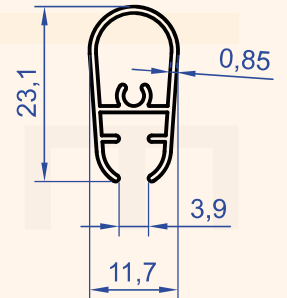
Profil No : 2022 Gramaj : 0.168 kg/m
