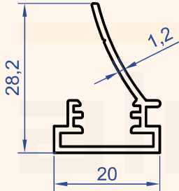
Profil No : 1042 Gramaj : 0.240 kg/m
