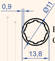
Profil No : 1042 Gramaj : 0.240 kg/m
