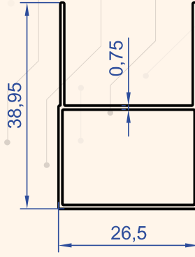
Profil No : 2133 Gramaj : 0.259 kg/m
